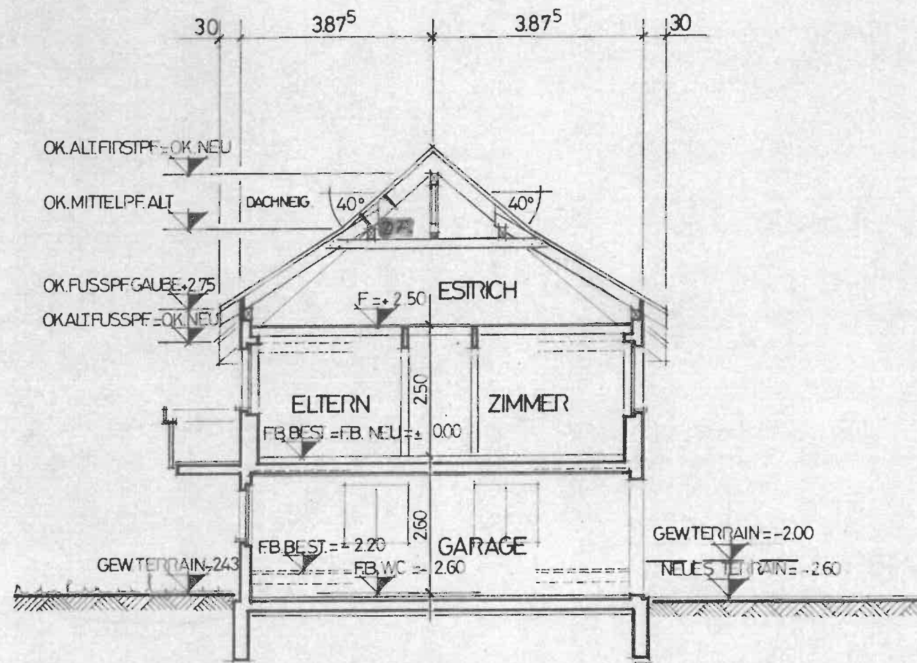
SCHNITT A-A
